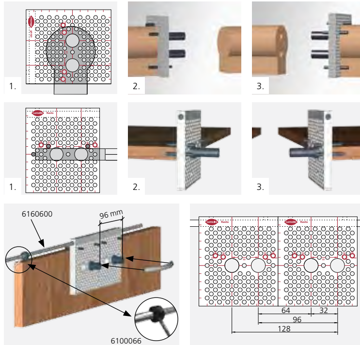
Borings voor handgrepen en rijborings in 32 mm raster
